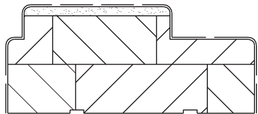
RJ-04 Wrapped Veneer Jamb
