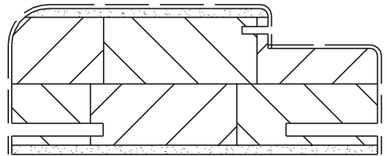
RJ-02 Wrapped Veneer Jamb
