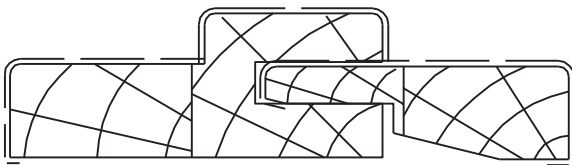
SJ-01 Split Jamb
