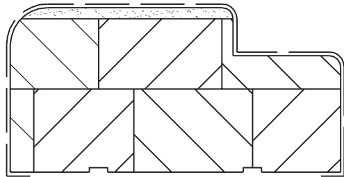
RJ-03 Wrapped Veneer Jamb
